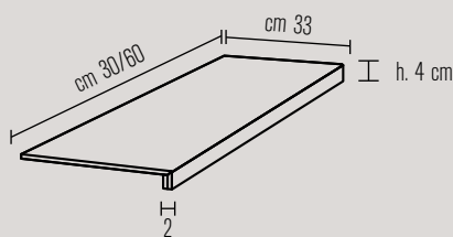
gradone (assemblato)
