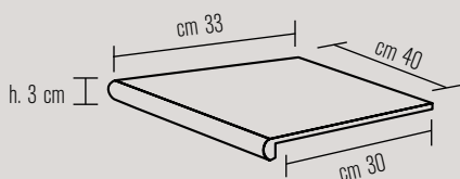
scalino
