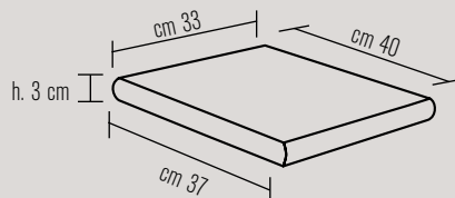
scalino angolare
