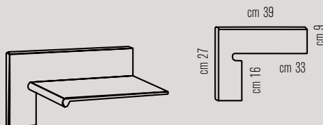
battiscala sx**
